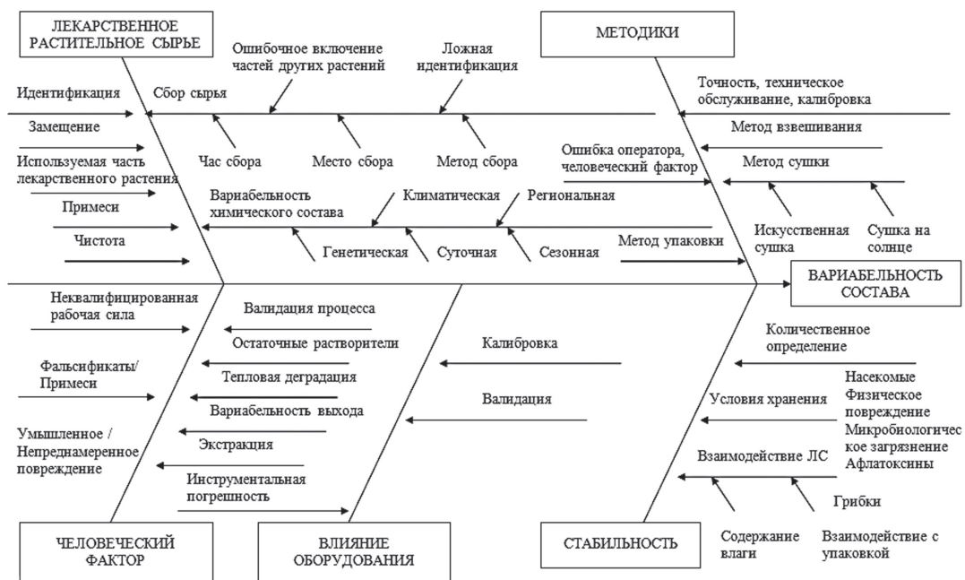
Рис. 1. Причинно-следственная диаграмма вариабельности растительных препаратов
