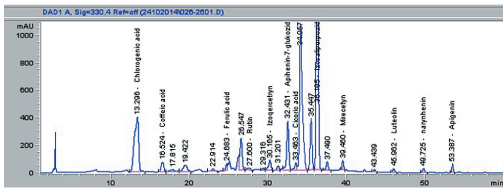
Рис. 5. Типова хроматограма випробовуваного розчину квіток цмину піскового ( Helichrysum areнарium L.), отримана під час ідентифікації флавоноїдів методом ВЕРХ
