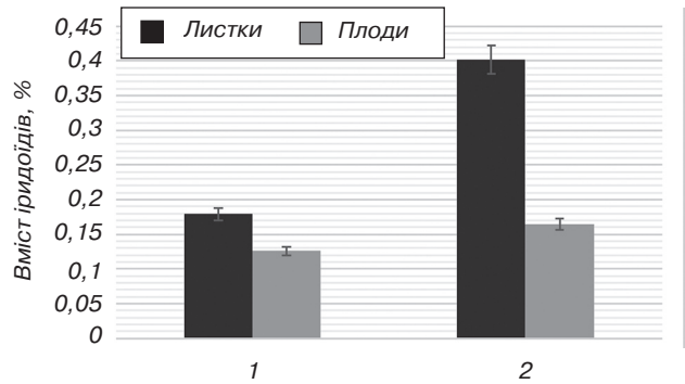
Рис. 3. Вміст іридоїдів у листках та плодах рослин: 1 — A. polygama та 2 — A. Macrosperma
