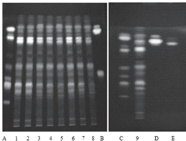
Рис. 4. Хроматограми порівняння розчинів, отриманих під час ідентифікації флавоноїдів у квітках цмину піскового методом ТШХ (знизу — вгору): А — рутин, хлорогенова кислота, гіперозид, апігеніну-7-глюкозид, ізосаліпурпозид, цикорієва кислота, лутеолін; В — лутеолін-7-глюкозид, кофейна кислота, кверцетин; С — рутин, хлорогенова кислота, гіперозид, апігеніну-7-глюкозид, ізосаліпурпозид, цикорієва кислота, лутеолін, апігенін; D — кофейна кислота, кверцетин; Е — розмаринова кислота, ферулова кислота; 1–9 — зразки квіток цмину піскового із досліджуваних спиртових витягів
