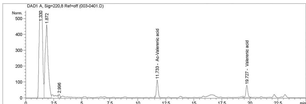
Рис. 1. Хроматограма з визначення суми сесквітерпенових кислот (ацетоксивалеренова + валеренова кислоти) в сировині з рівнем передполивної вологості ґрунту (РПВr) 70%
